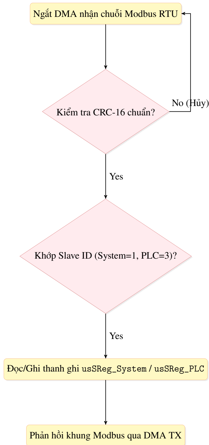
Hình 4.7 Sơ đồ luồng xử lý giao thức Modbus RTU trên các cổng truyền thông.
