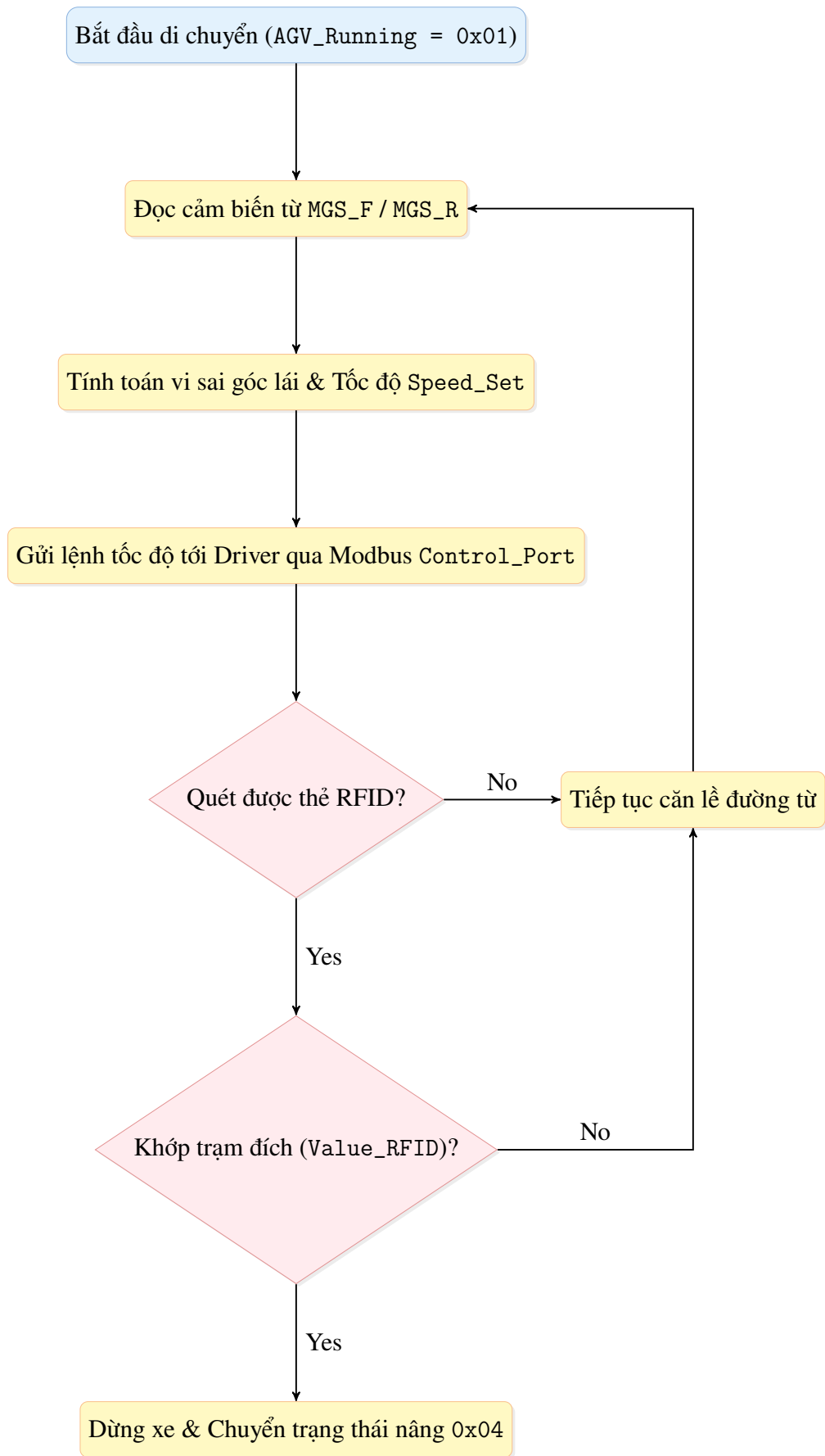
Hình 4.3 Sơ đồ thuật toán dẫn đường từ và định vị vị trí trạm bằng thẻ RFID.
