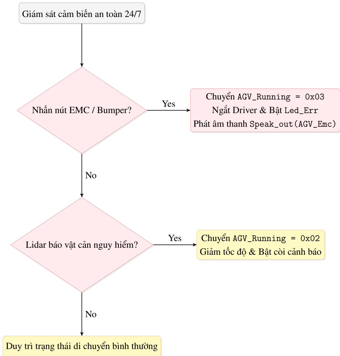
Hình 4.4 Sơ đồ tuần tự xử lý an toàn Lidar, Bumper và Nút khẩn cấp.
